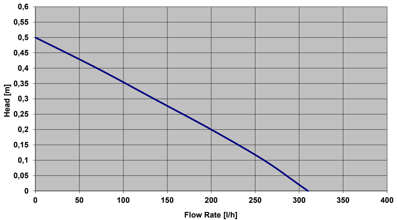
MI MOUSE - Kennlinie
