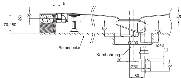
Darstellung mit Ablaufgarnitur - 0,6 l/s, senkrechte Entwässerung
