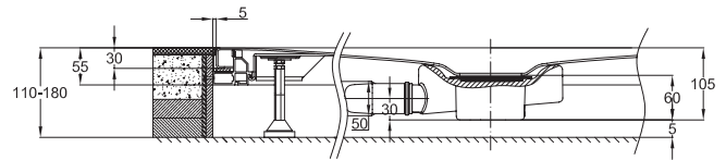
Darstellung mit Ablaufgarnitur BETTEFLOOR - 0,85 l/s, seitlicher Entwässerung
